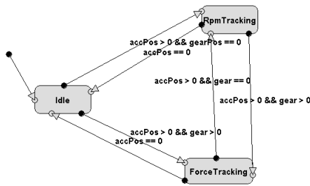
Abbildung 4: MSD für EngineController für je nach Wertbelegung der Eingänge gear (eingeleger Gang) und accPos (Gaspedalstellung) umgeschaltet.
